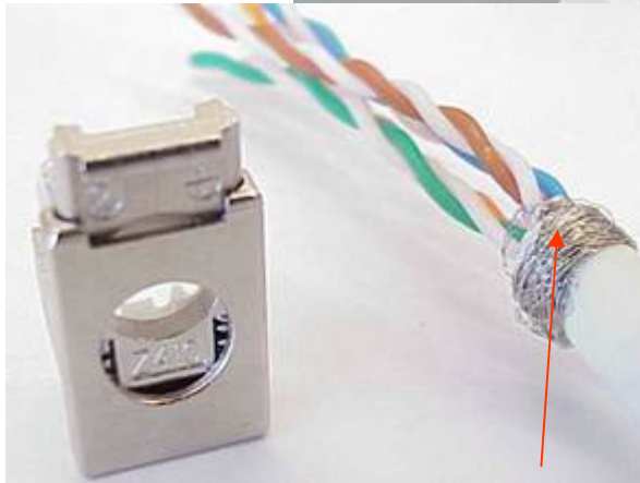
Tresse blindage
