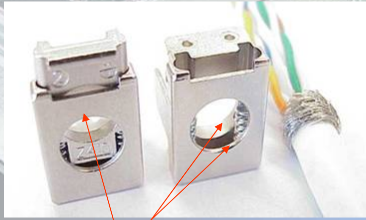
3 surfaces métalliques en contact avec la tresse de masse du câble
